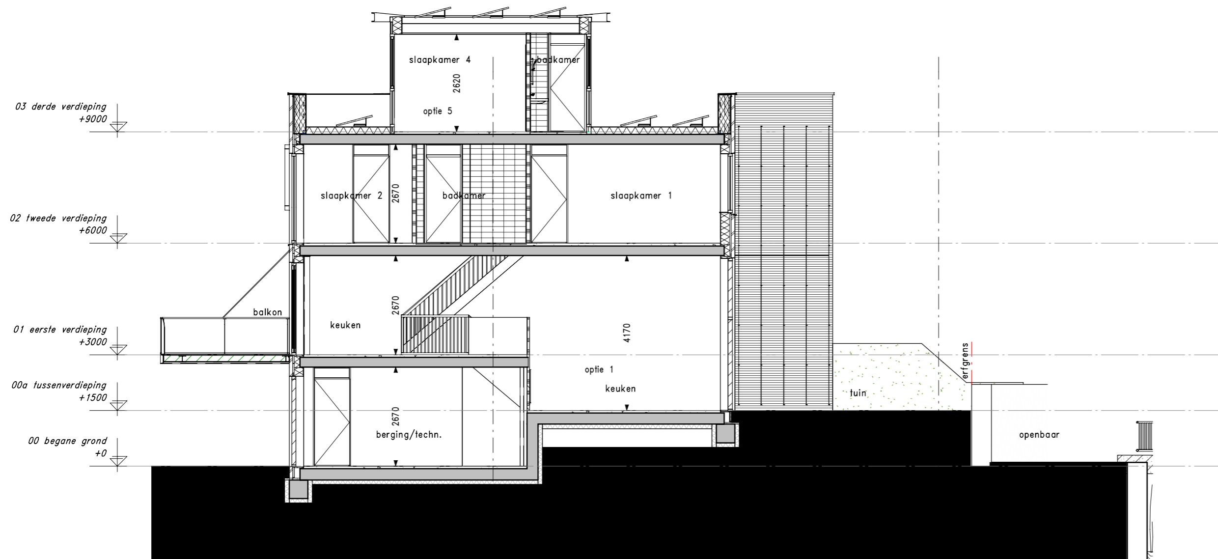
Doorsnede A-A (optie 1 en 5)
