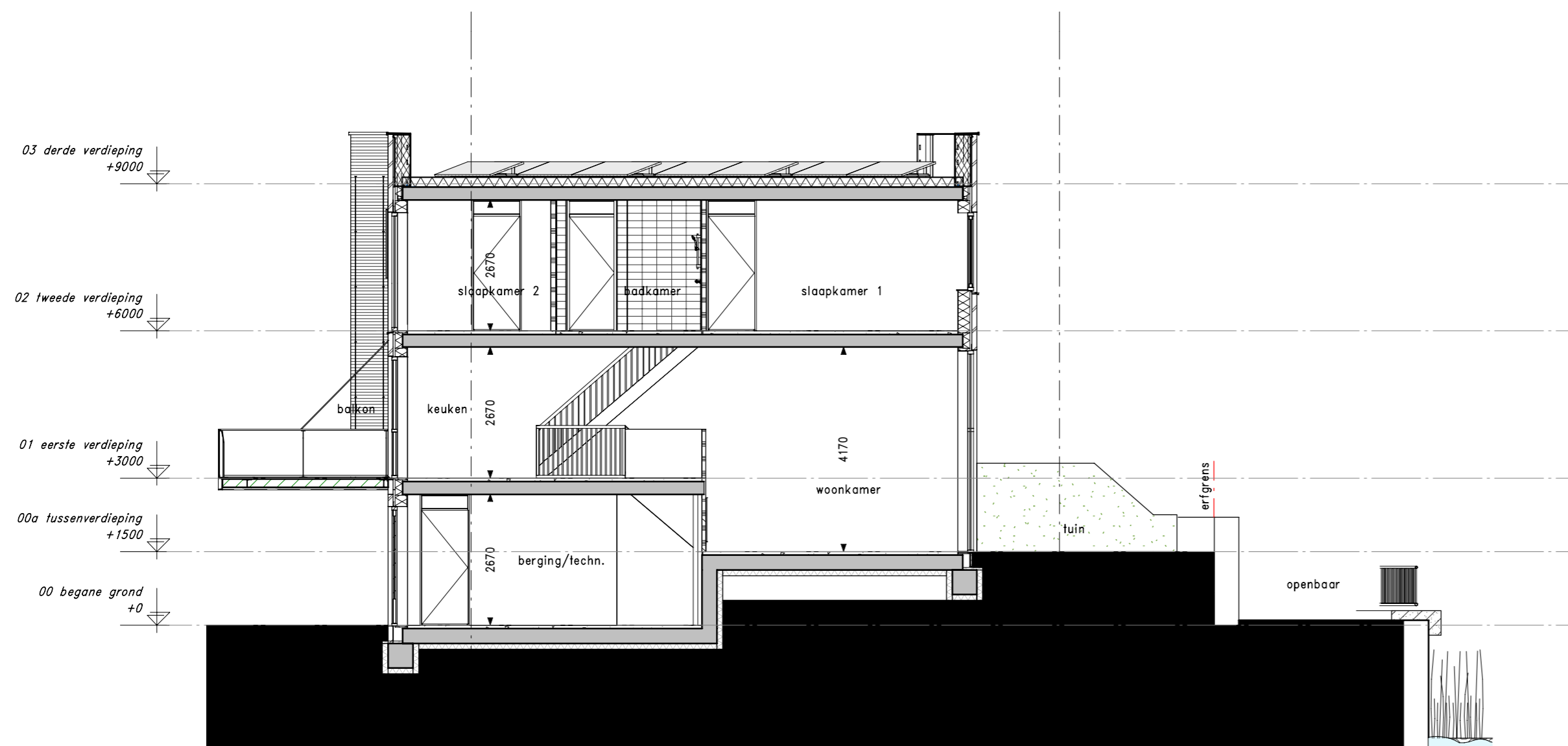
Doorsnede A-A
