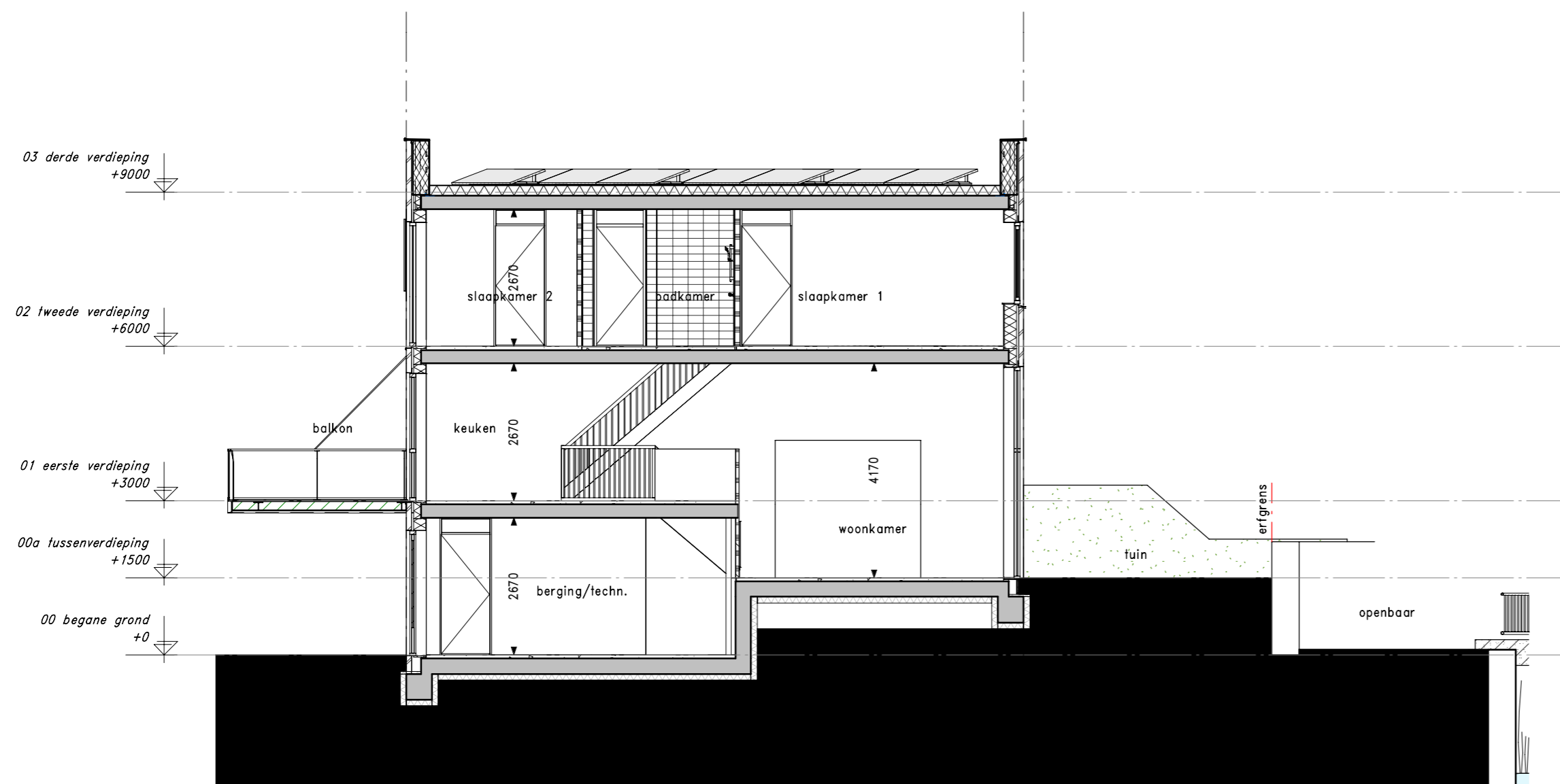
Doorsnede A-A
