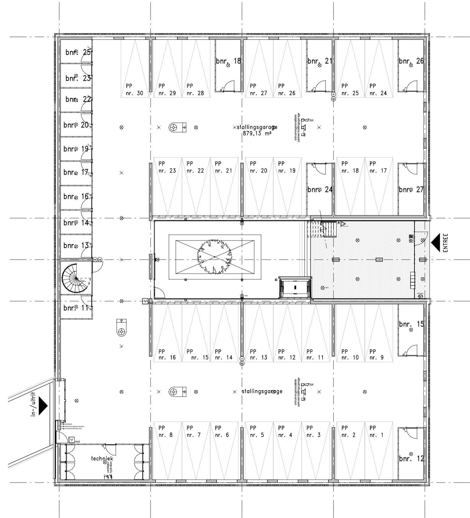
Kelder/Begane grond
