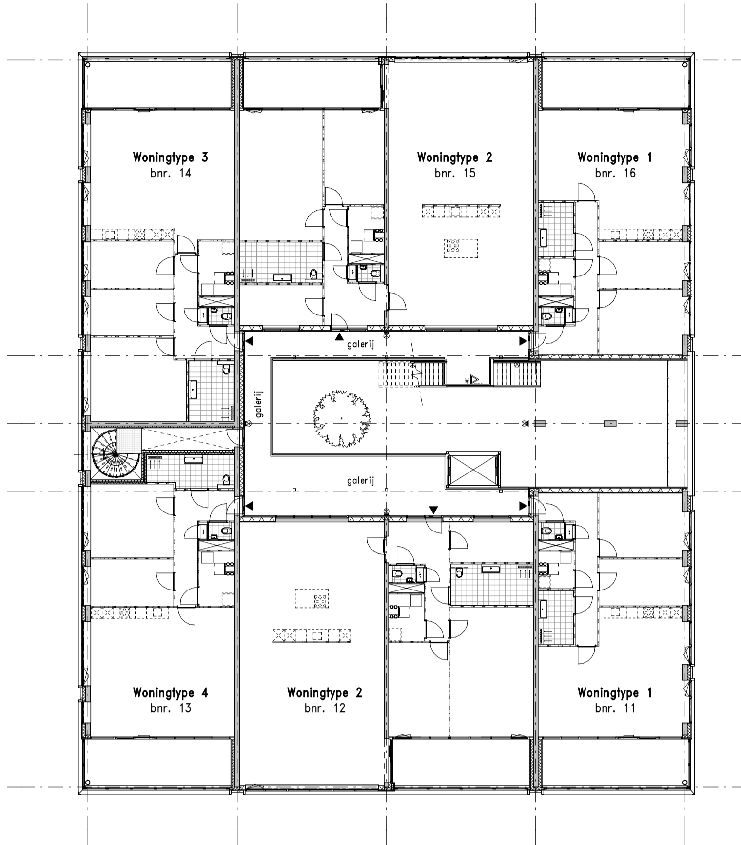
1e verdieping
