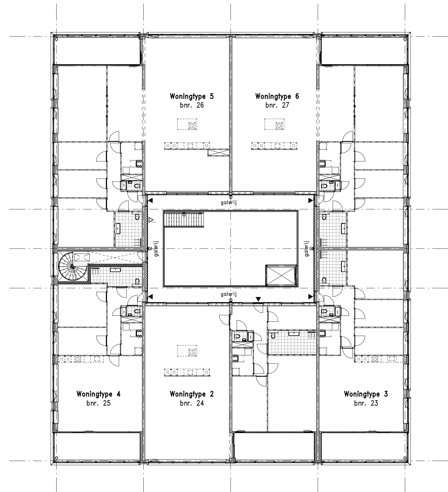
3e verdieping
