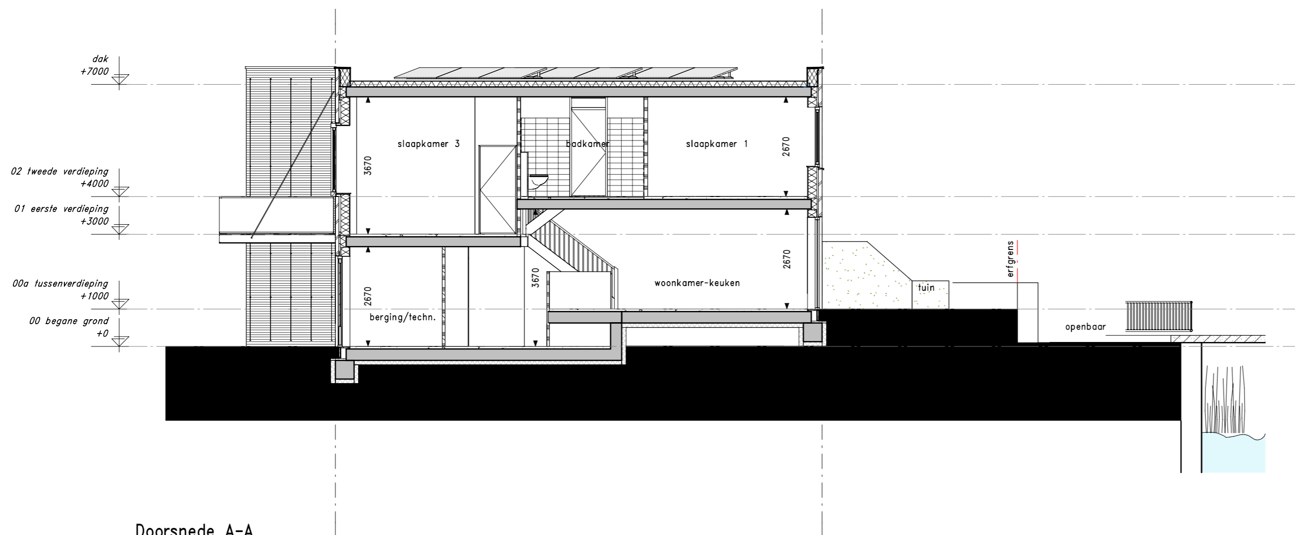
Doorsnede A-A
