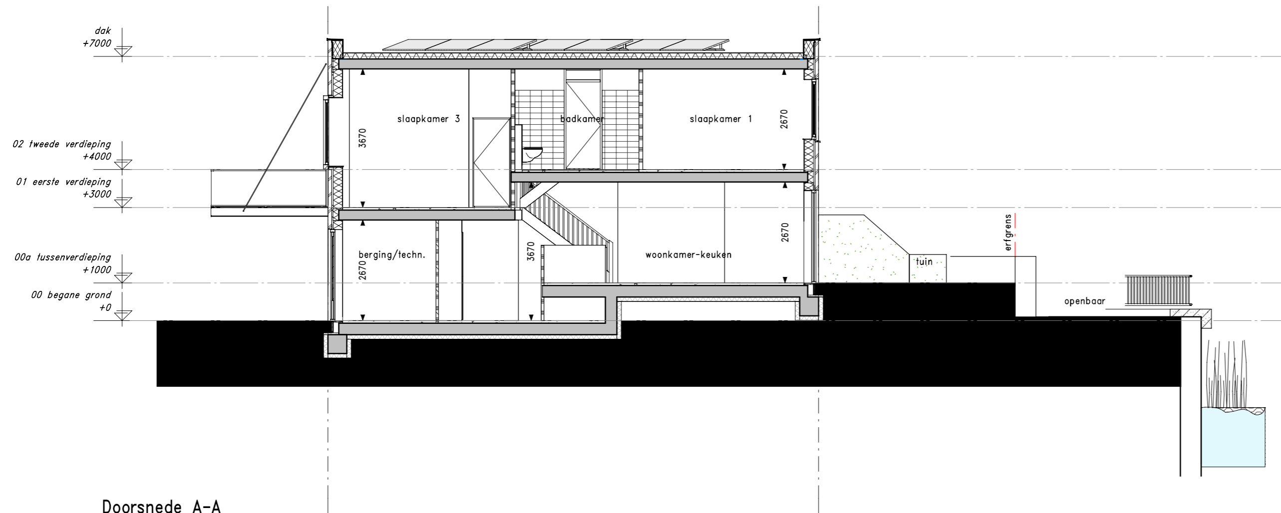
Doorsnede A-A
